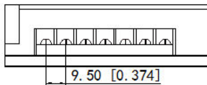
前视图 Frontview
