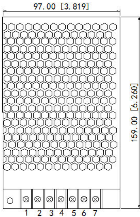
顶视图 Topview
